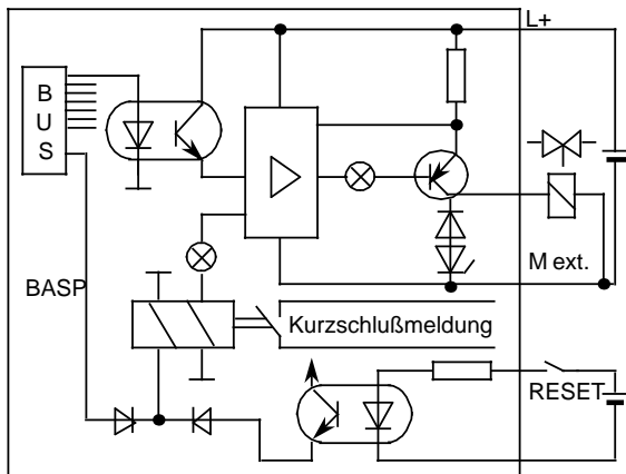
Principalschaltbild
