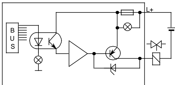
Principalschaltbild
