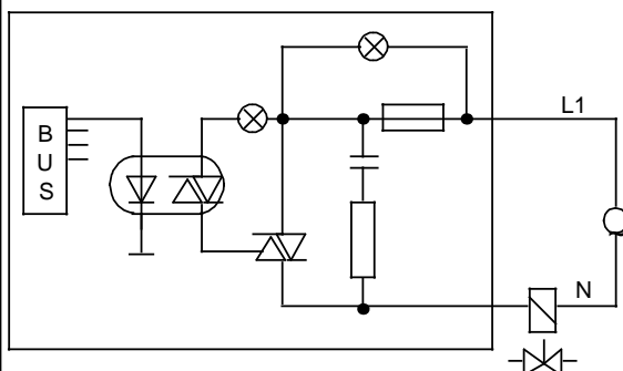
Prinzipialschaltbild
