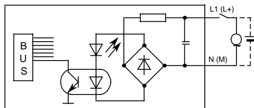
Prinzipschaltbild
