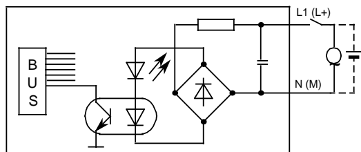
Prinzipschaltbild
