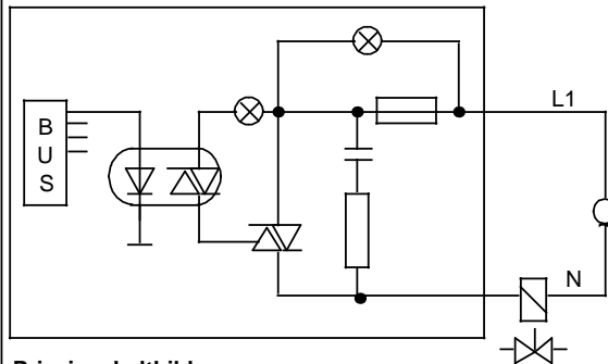
Prinzipschaltbild
