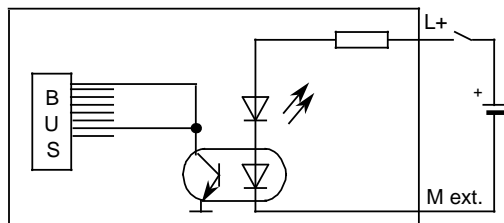
Prinzipschaltbild
