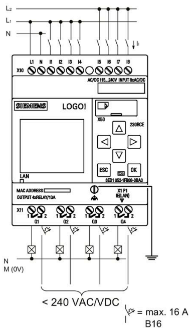
Zweiphasige Verbindung des Basismoduls
