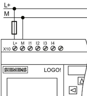
LOGO! ... mit DC-Versorgung
