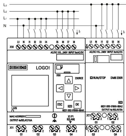
Dreiphasige Verbindung des Basismoduls mit einem Erweiterungsmodul
