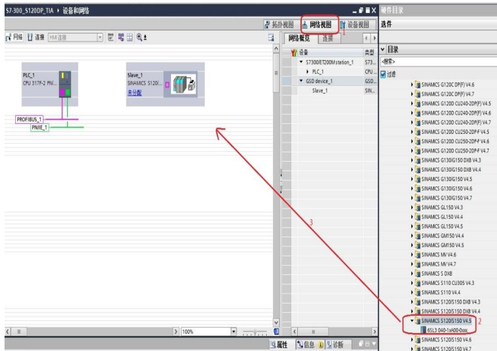
图 3-4 硬件组态
