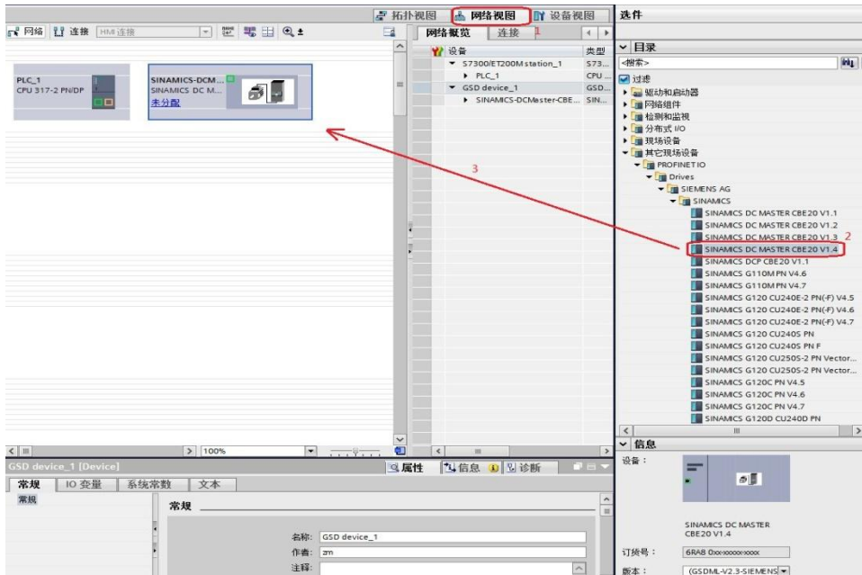
图 3-2 硬件组态
