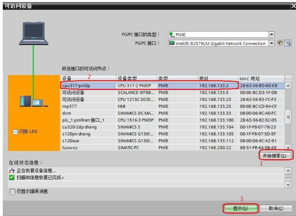
图 3-5 搜索节点
