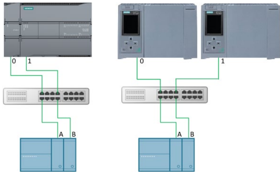
图 13-14 双侧冗余
