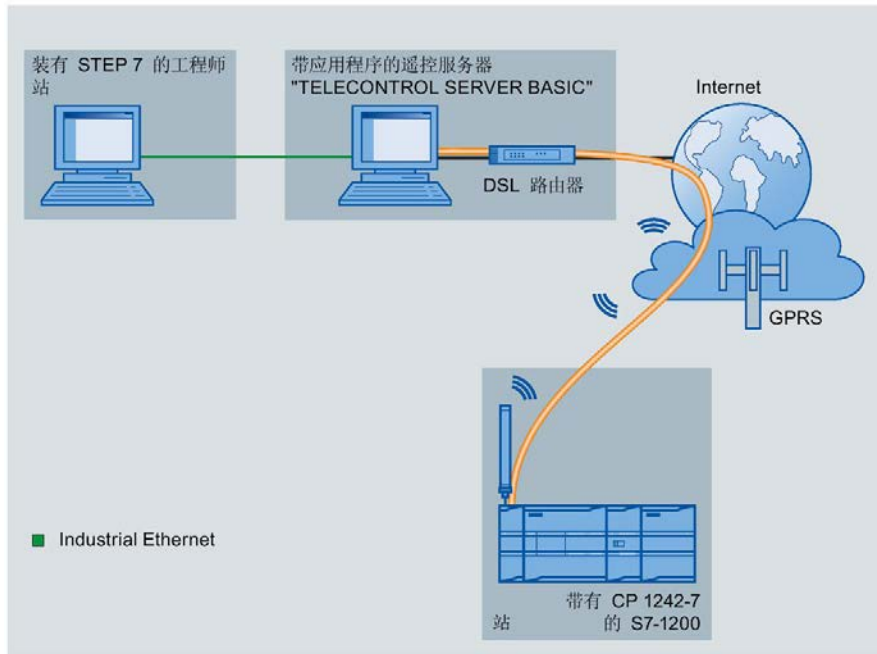
图 13-31 在使用遥控服务器的组态中通过 GPRS 的 TeleService
