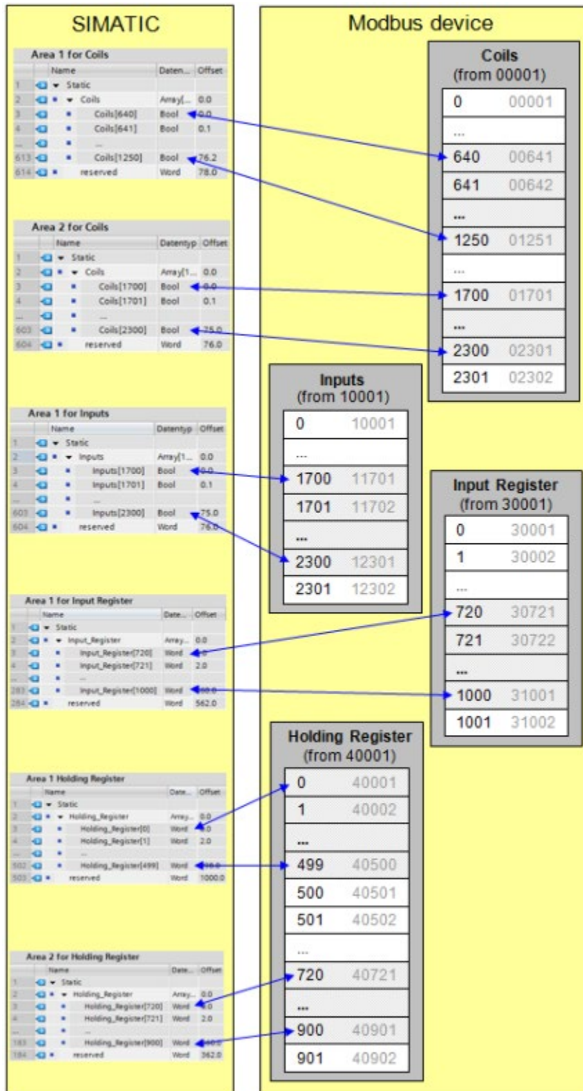
图 13-23 地址构建
