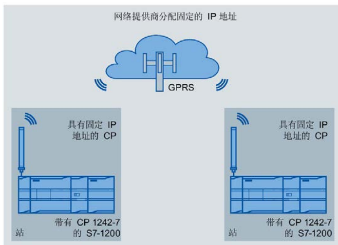
图 13-30 两个 S7-1200 站间直接通信
