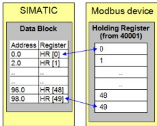
图 13-27 MB_HOLD_REG: 偏移量为 0 的数据块
