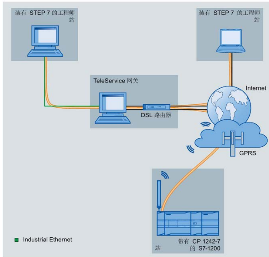
图 13-32 在使用 TeleService 网关的组态中通过 GPRS 的 TeleService
