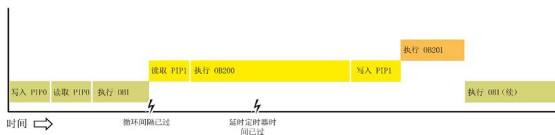
图 5-1 情况 1：不可中断 OB 执行
