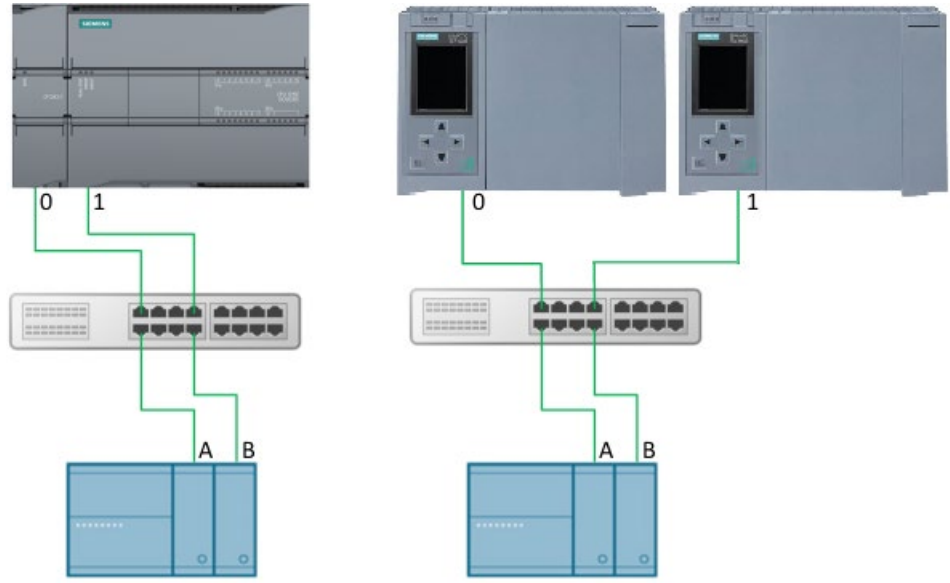
图 13-3 双侧冗余
