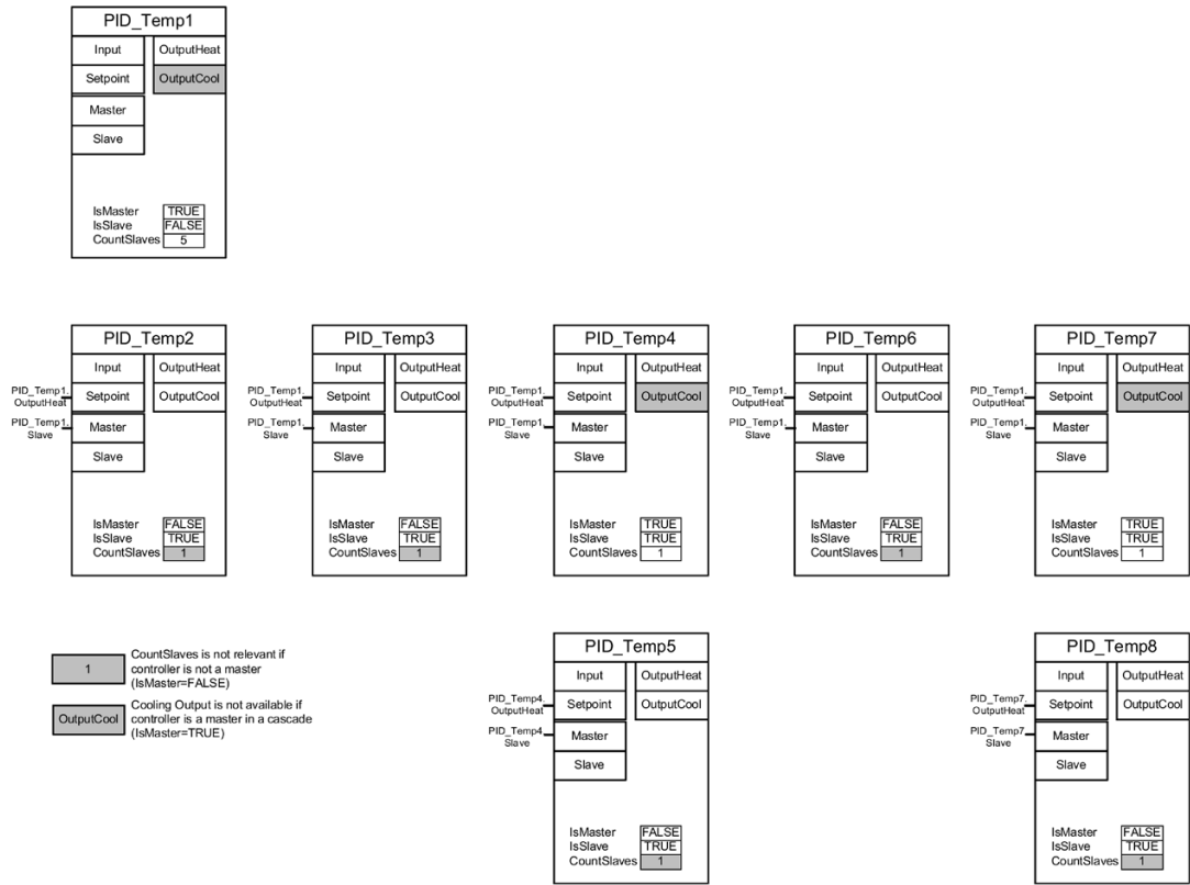
图 10-8 PID_Temp_Cascading_communication_connection
