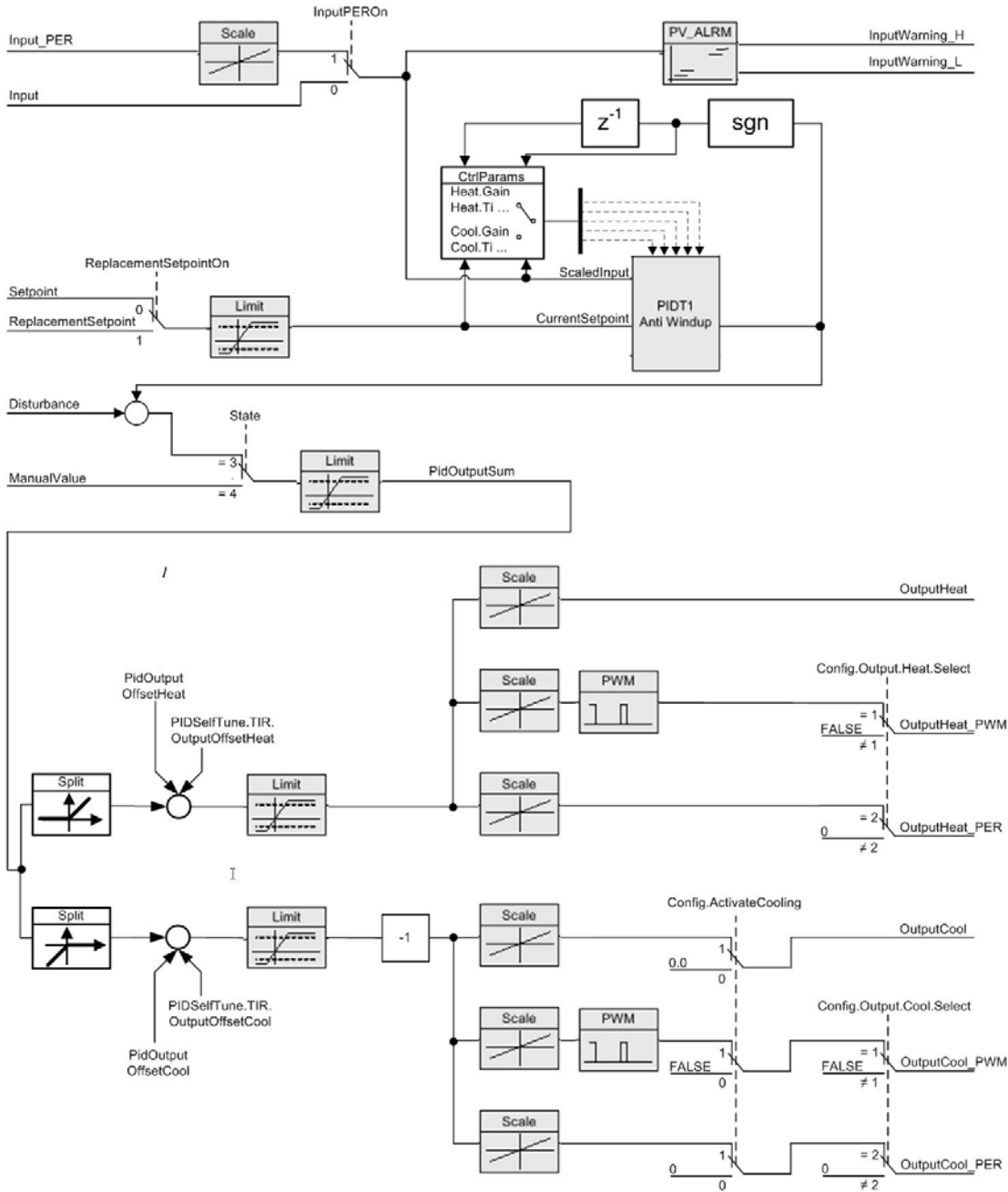
图 10-6 PID_Temp_Operation_Block_Diagram
