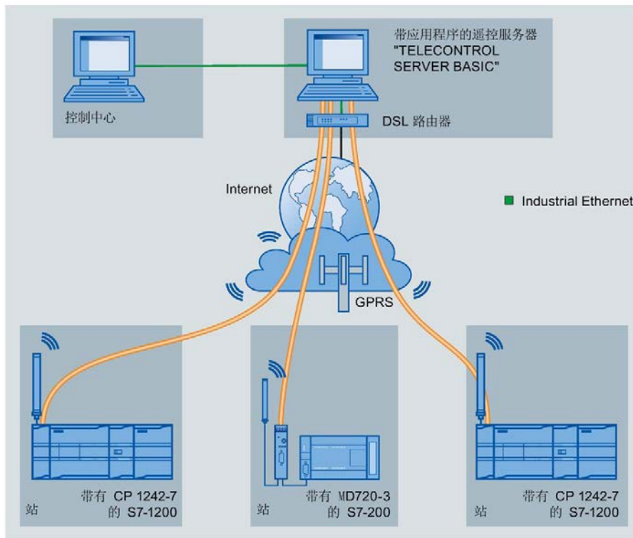
图 13-29 S7-1200 站与控制中心之间的通信
