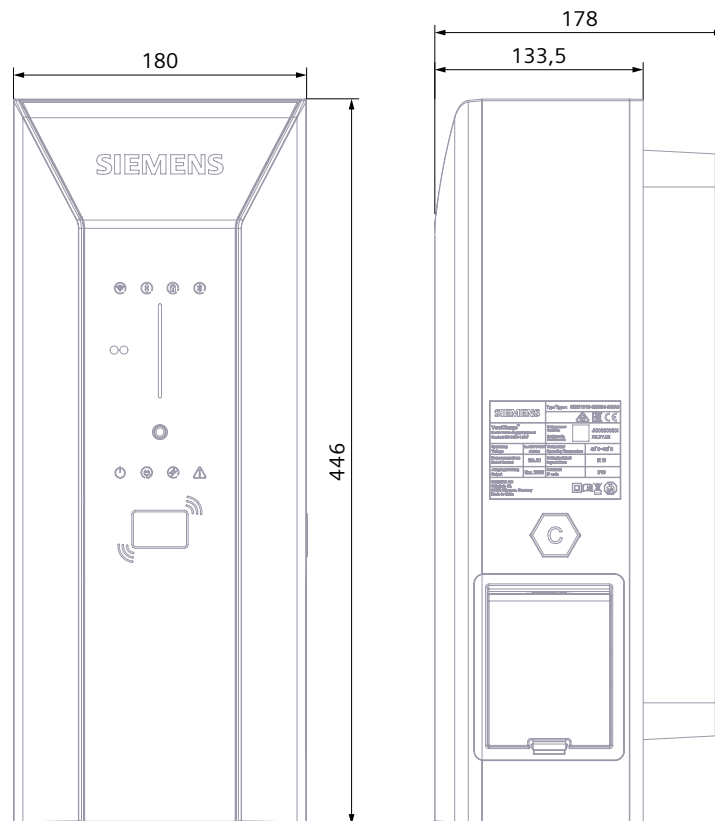
Bild A-1 Maßbild der Wallbox
