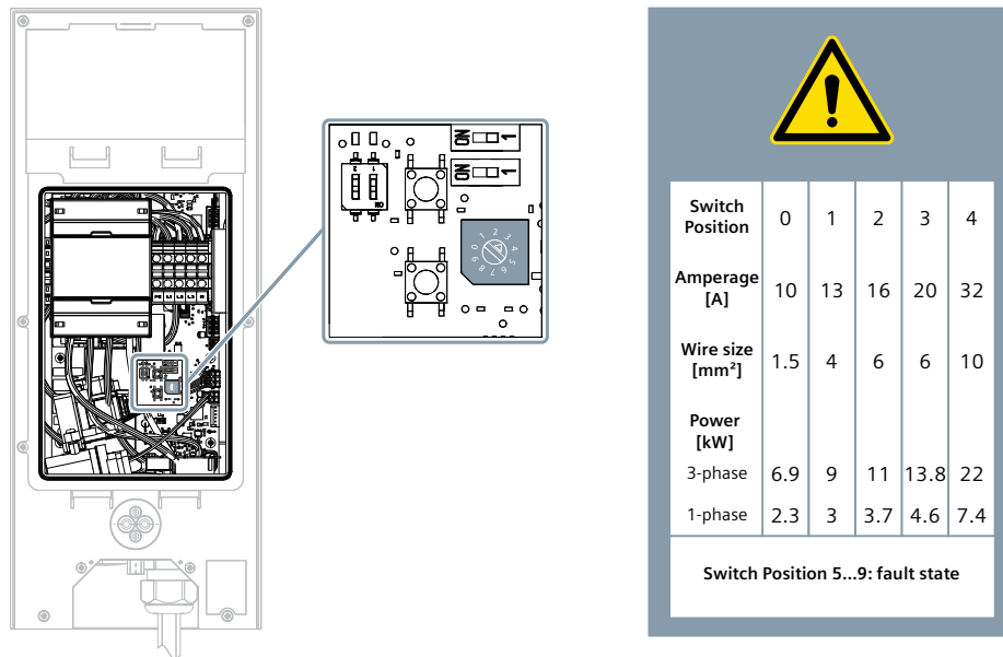
Bild 4-6 Ladestrom
