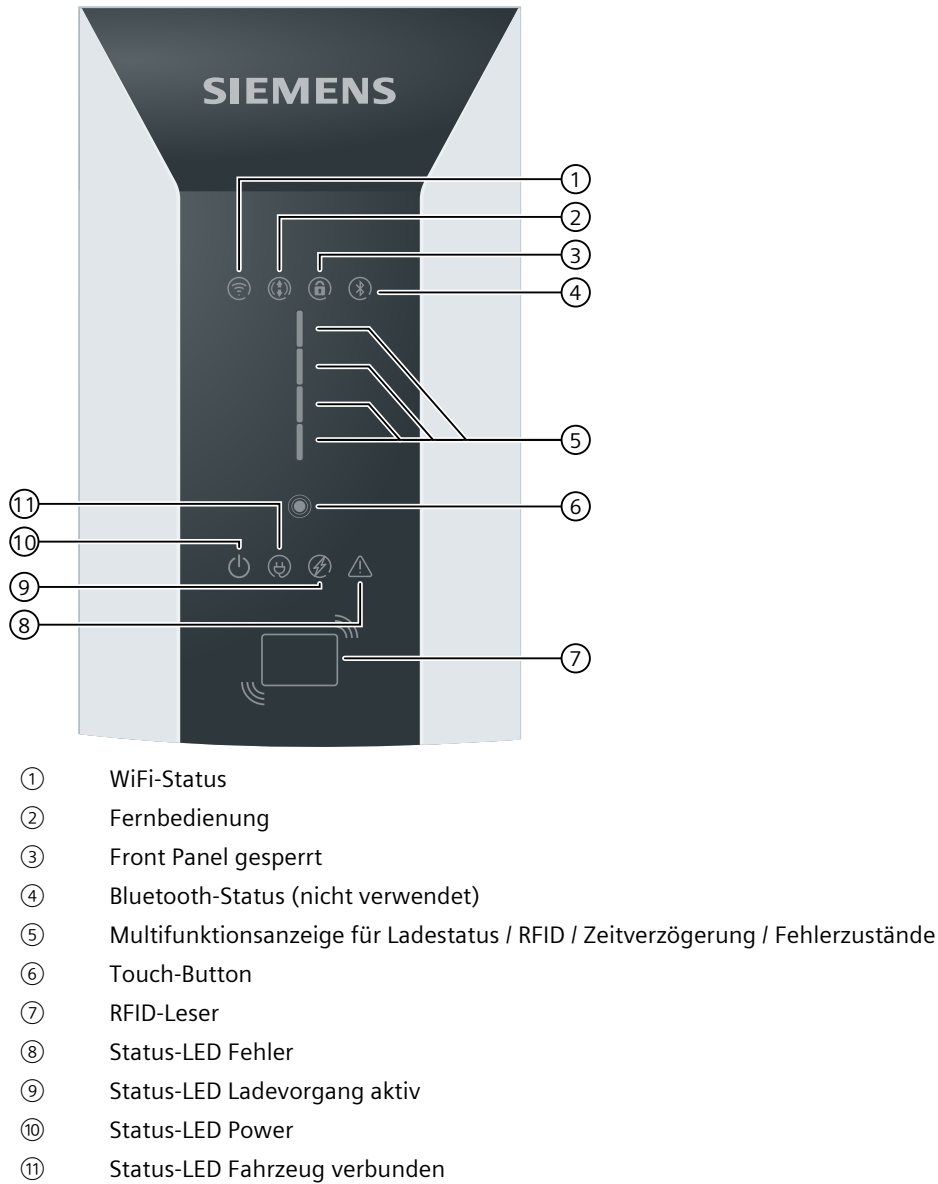
Bild 3-2 Aufbau der Wallbox
