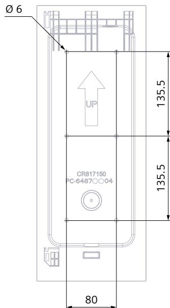
Bild 4-2 Bohr Bild
