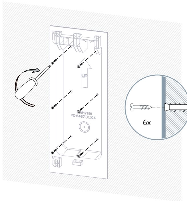
Bild 4-3 Wandhalterung montieren
