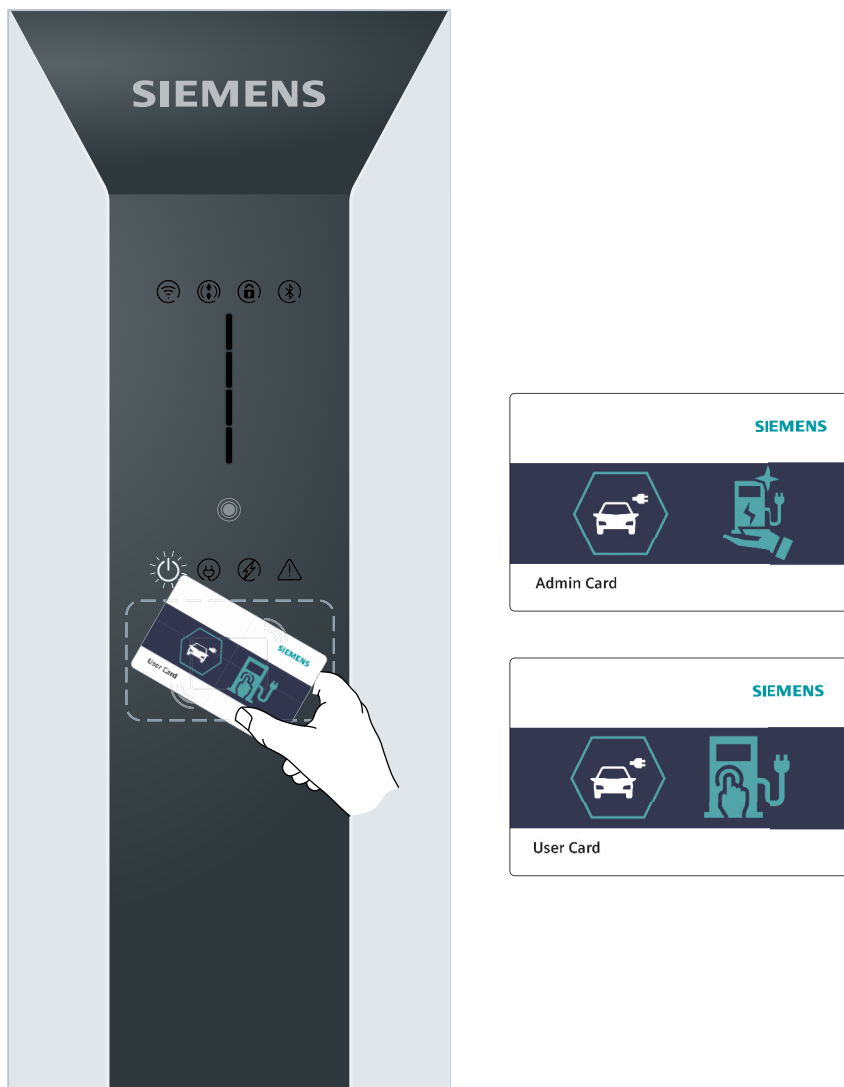
Bild 5-1 RFID-Kartentypen
