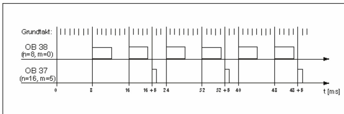
Priorität der Weckalarm-OBs
