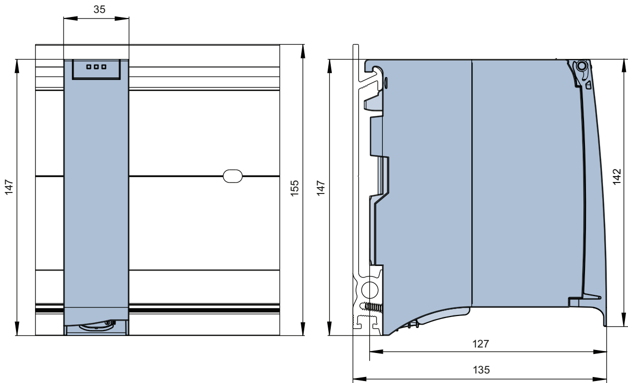
Bild A-1 Maßbild des Kommunikationsmoduls CM PtP RS232 HF
