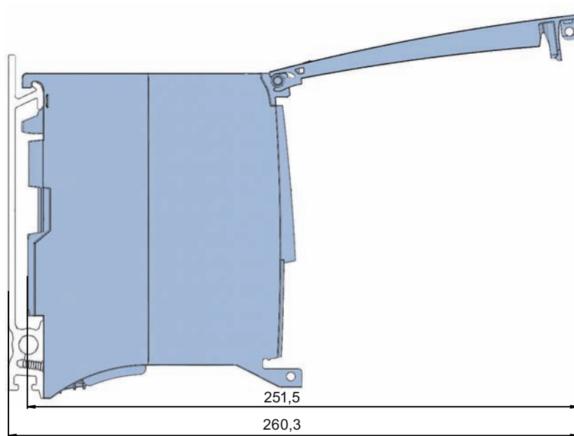
Bild A-2 Maßbild des Kommunikationsmoduls CM PtP RS232 HF mit geöffneter Frontklappe
