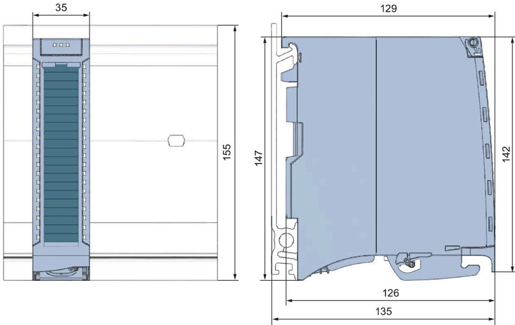
Figure A-1 Dimensional drawing of the DI 32x24VDC HF module
