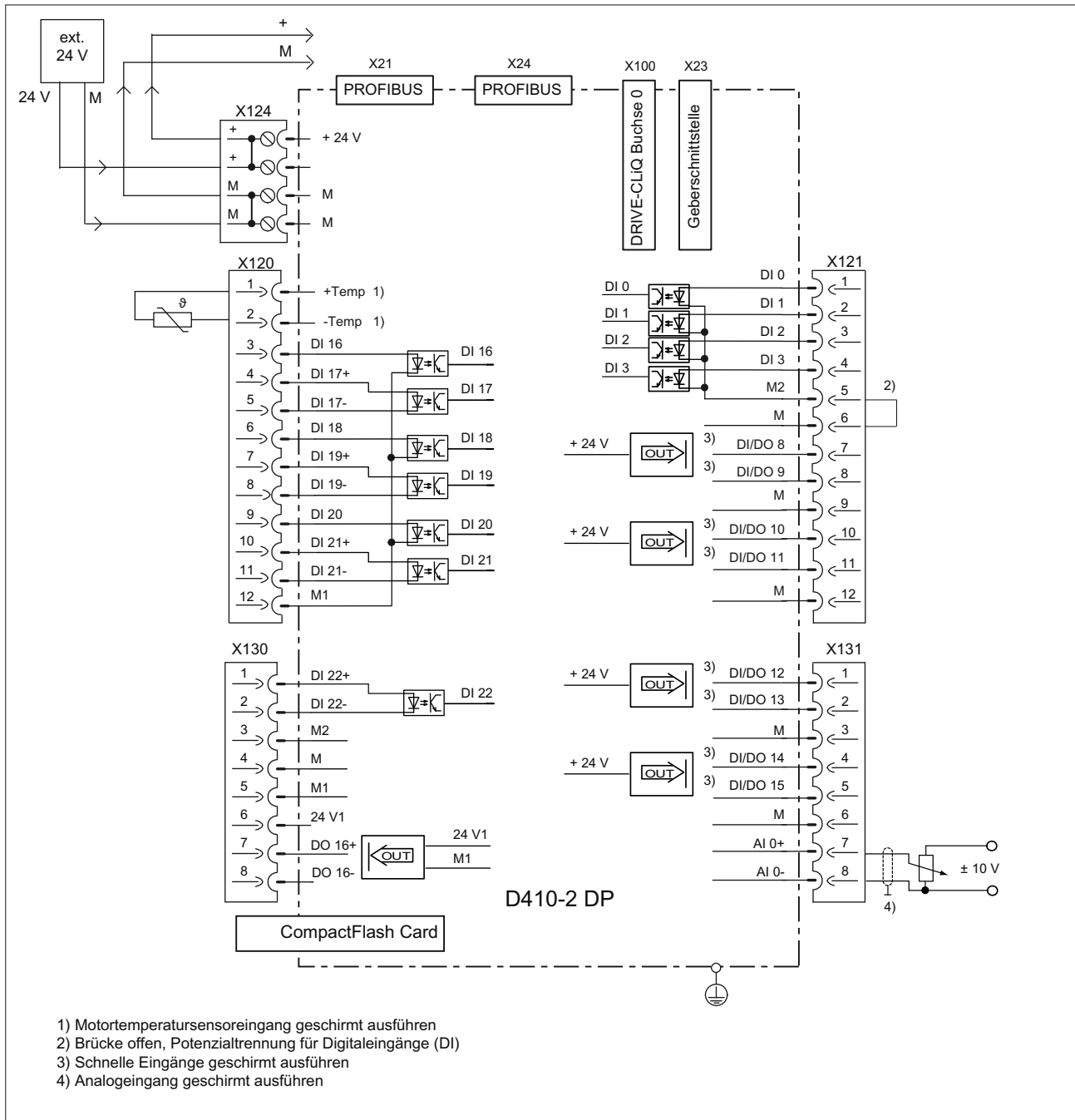
Bild 3-3 Innenschaltung der SIMOTION D410-2 DP ohne Safety-Funktion
