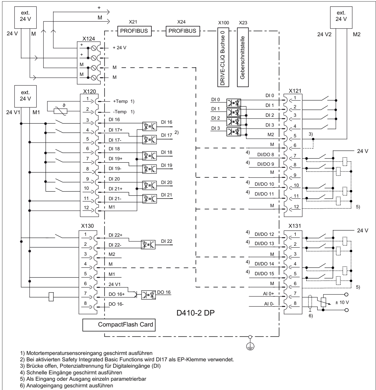
Bild 3-1 Anschlussbeispiel SIMOTION D410-2 DP
