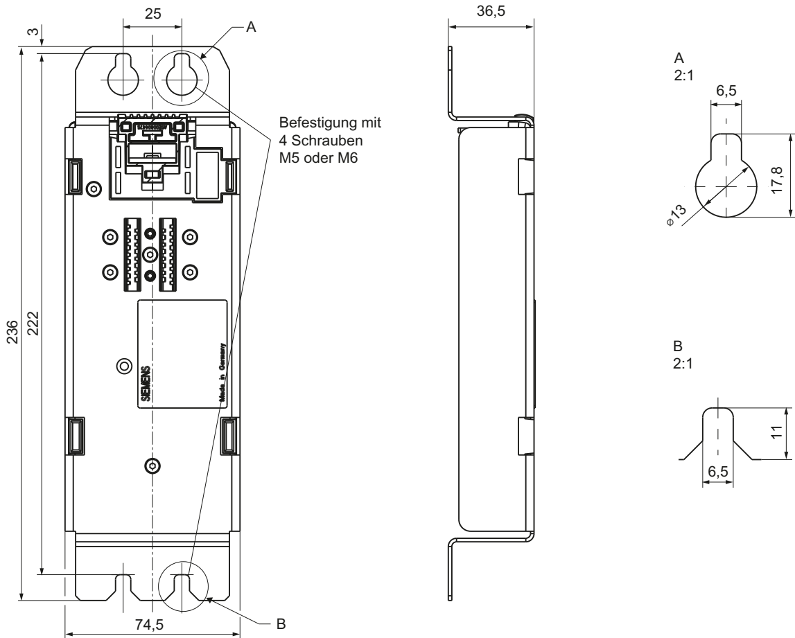
Bild 5-2 Maßbild Montageplatte
