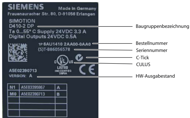
Bild 1-6 Typenschild SIMOTION D410-2 DP
