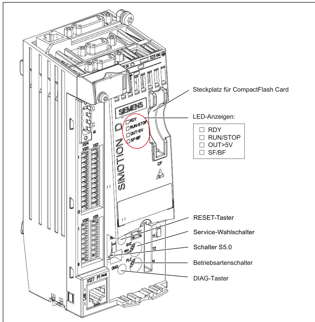
Bild 2-1 Bedien- und Anzeigeelemente SIMOTION D410-2
