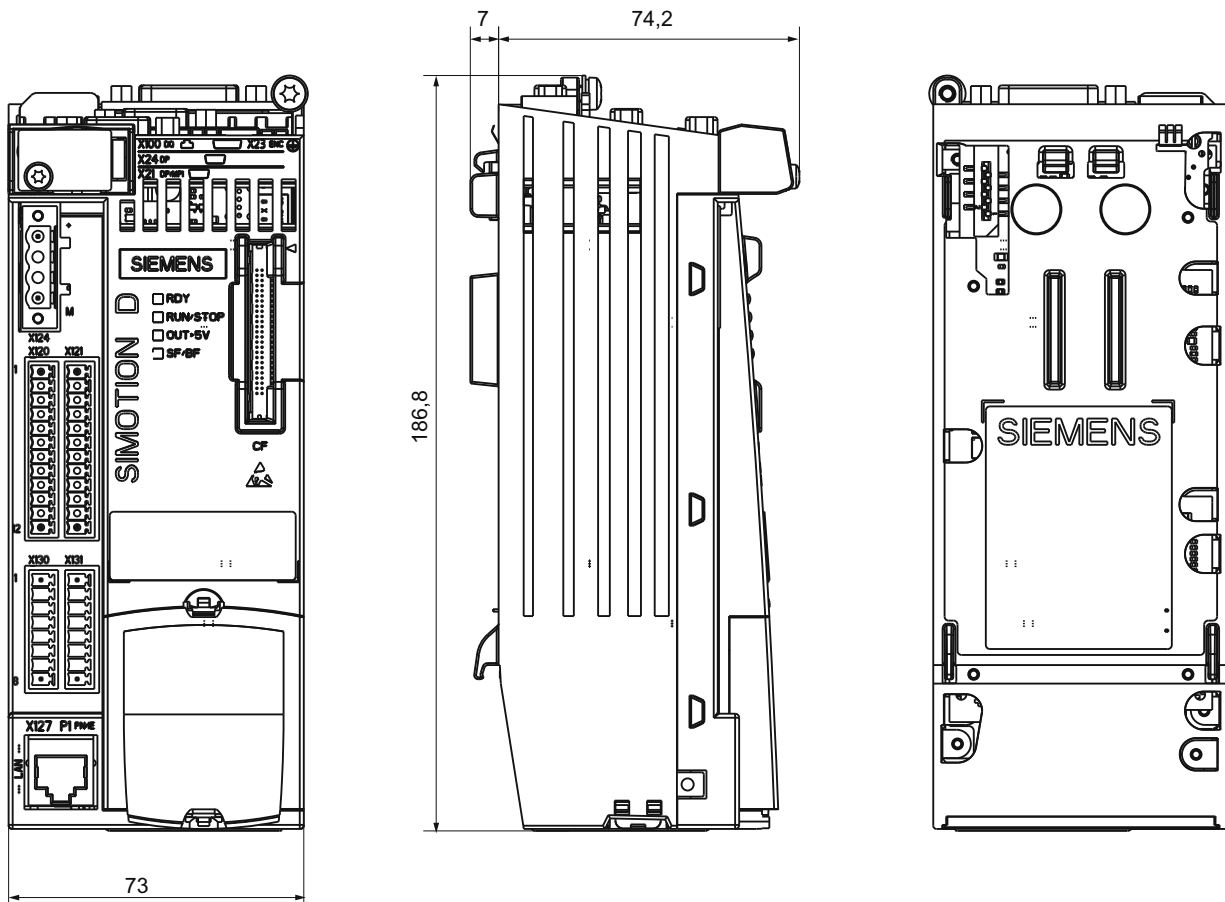
Bild 5-1 Maßbild SIMOTION D410-2 DP
