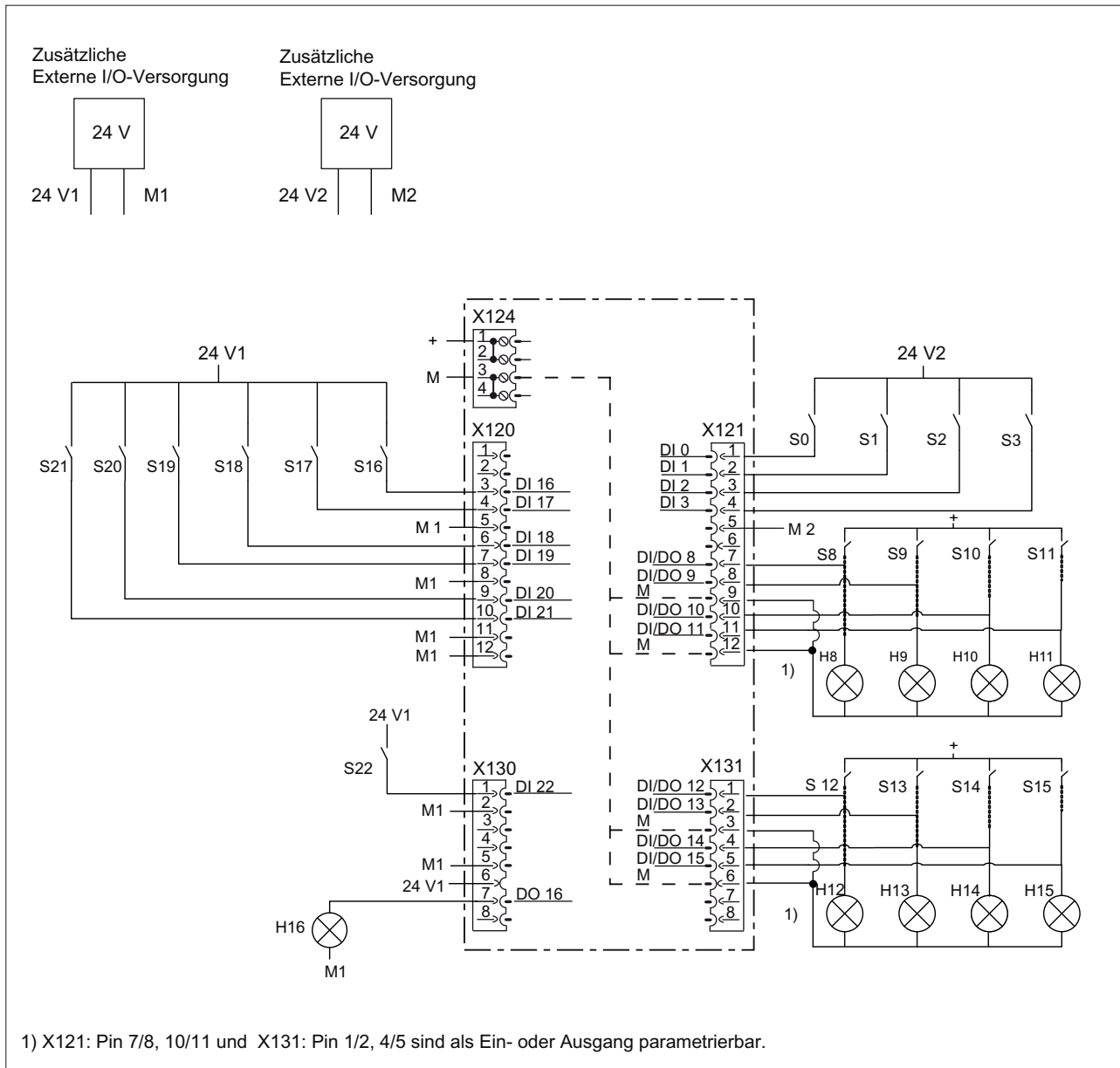
Bild 3-2 Beschaltungsbeispiel der DI / DO ohne Safety Funktion
