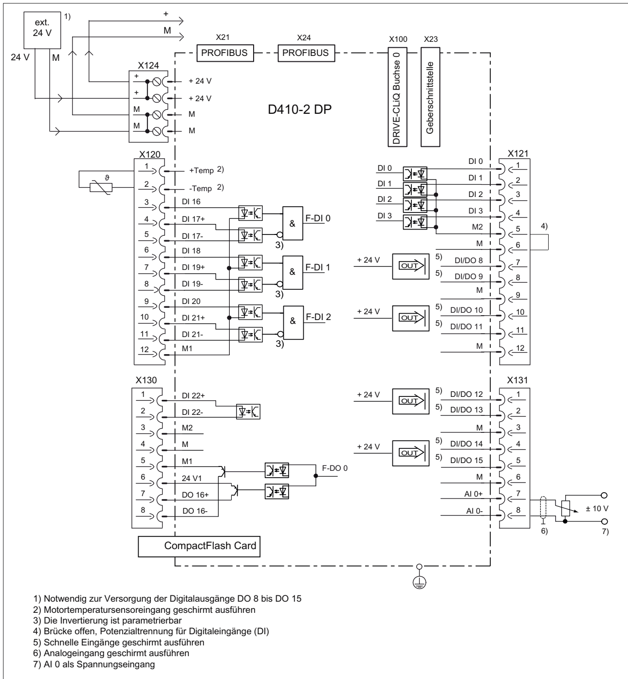
Bild 3-4 Innenschaltung der SIMOTION D410-2 DP mit Safety-Funktion
