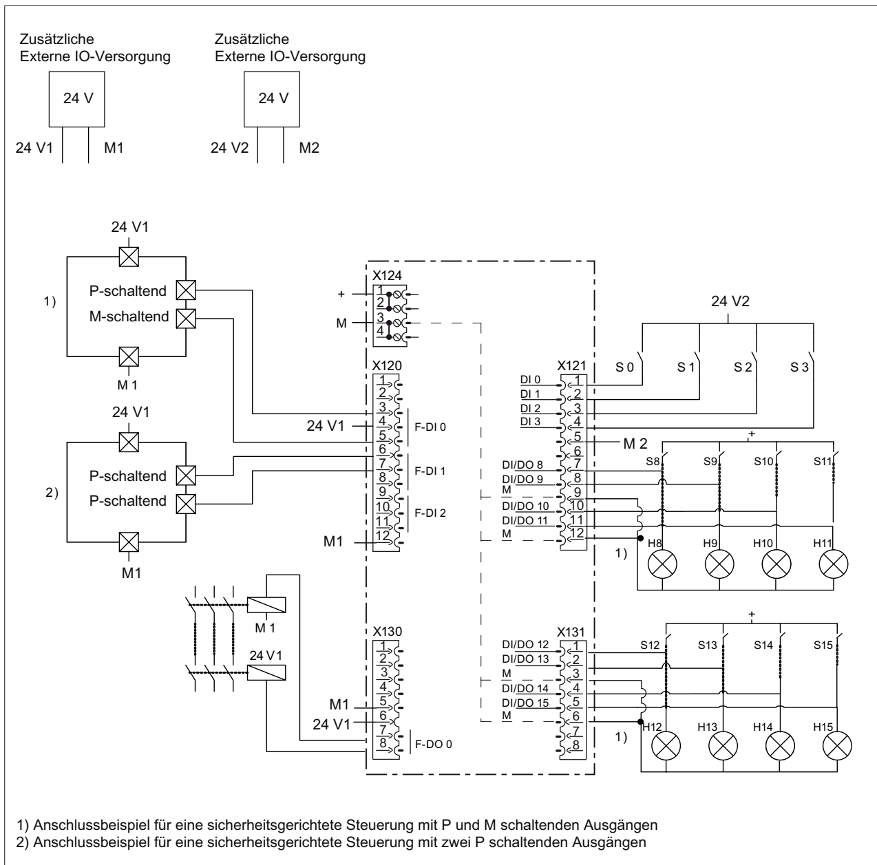
Bild 3-5 Beschriftungsbeispiel der F-DI und F-DO mit Safety Funktion
