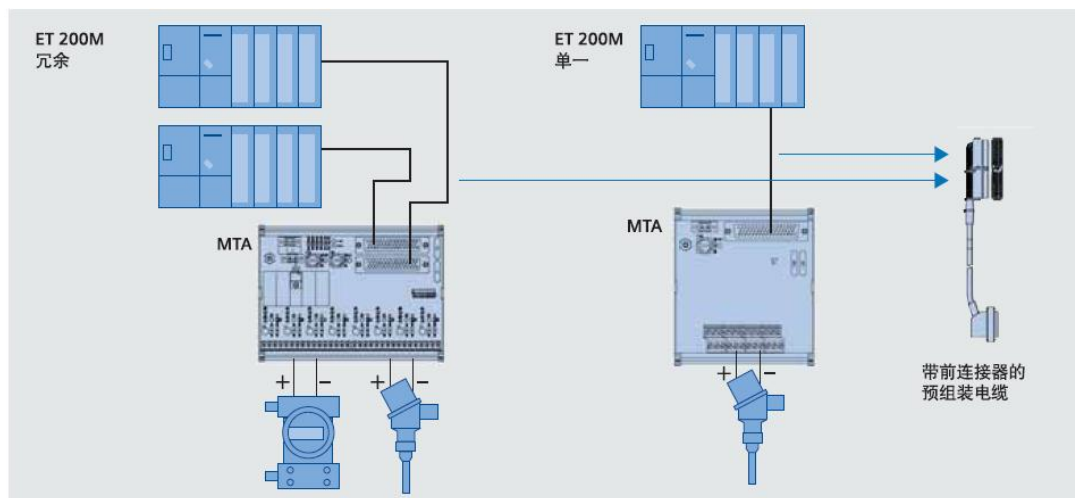
图 6 MTA 端子接线图例
