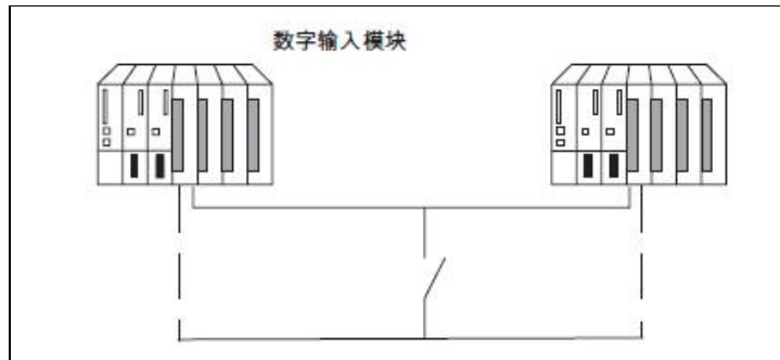
图 4 冗余数字量输入接线方式
