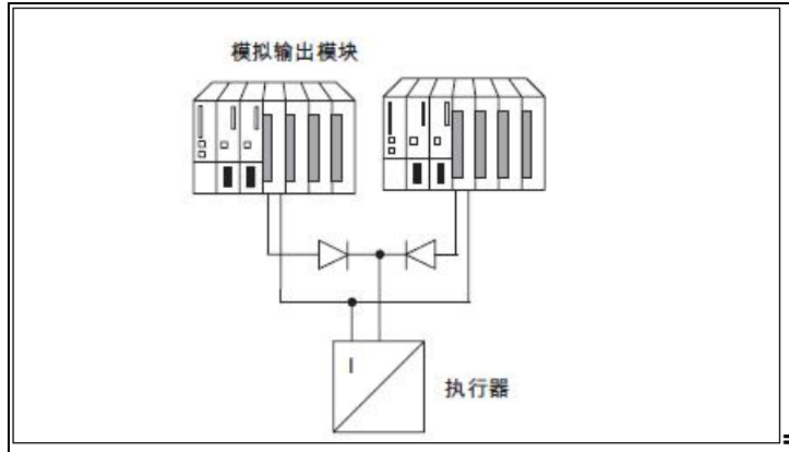
图 3 冗余模拟量输出接线方式
