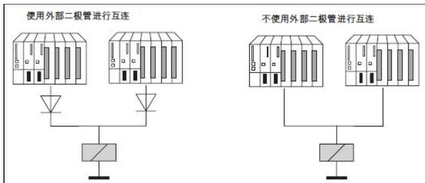
图 5 冗余数字量输出接线方式
