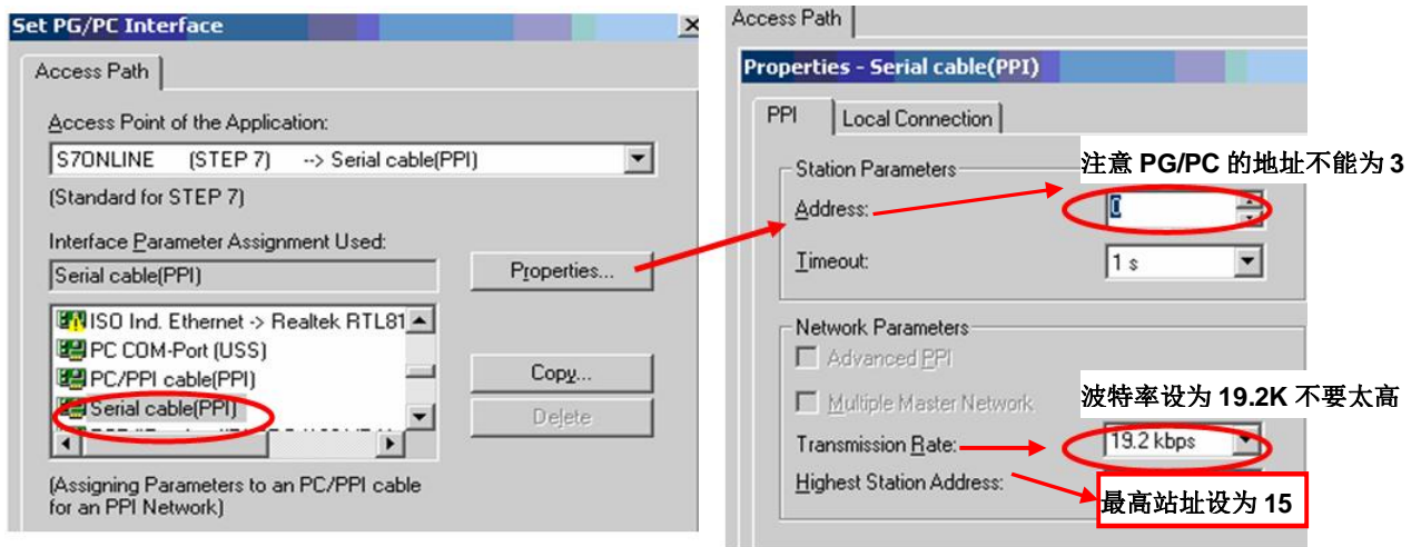
图 2 PG/PC 设置示意图
