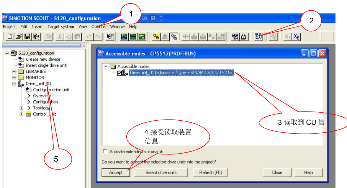
图 5 STARTER/SCOUT 自动搜索在线节点
