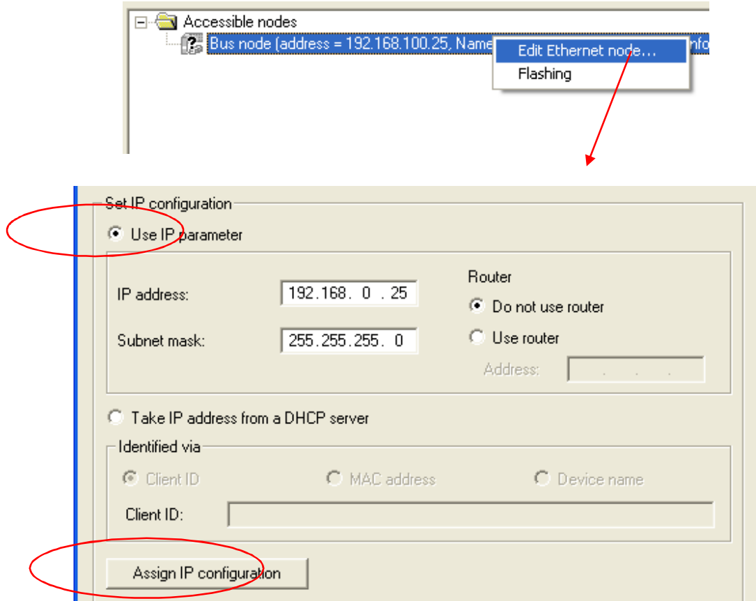
图 26 给在线节点分配 IP 地址
