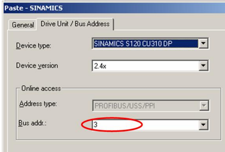
图 4 STARTER/SCOUT 中 S120 地址的设置
