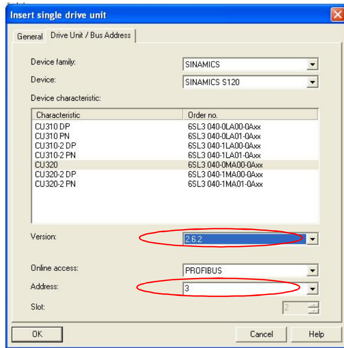
图 12 STARTER/SCOUT 中 DP 地址的设定
