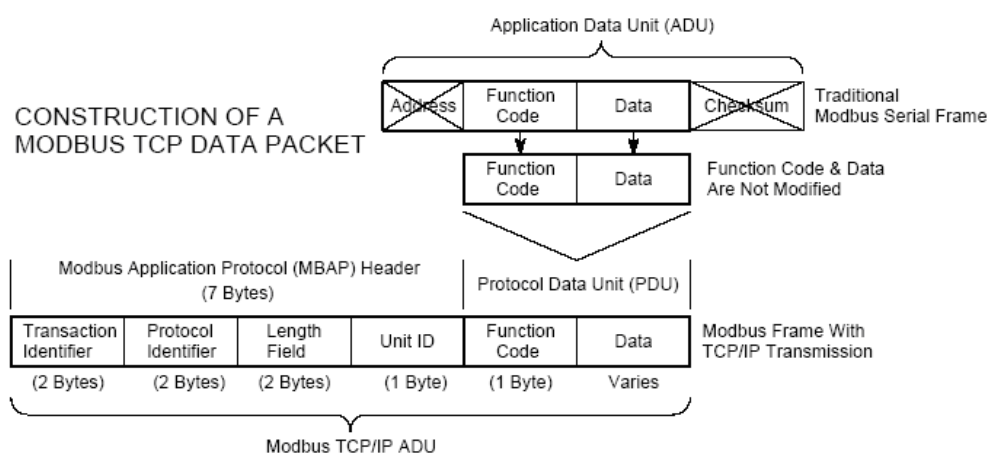
图 1: MODBUS TCP 报文
