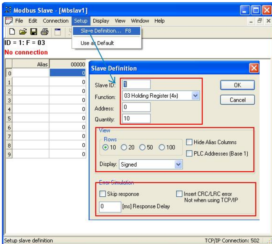
图 31: Modbus Slave 中 Modbus 数据参数定义
