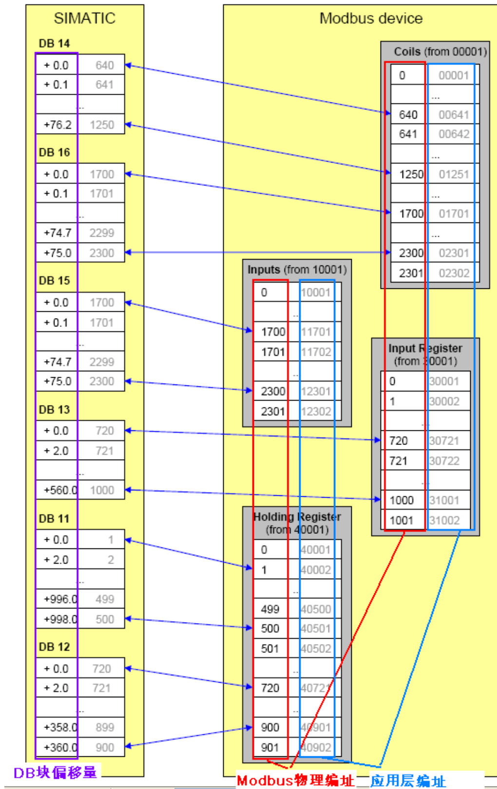
图 23: DB 偏移量、Modbus 物理编址、应用层编址对应关系
