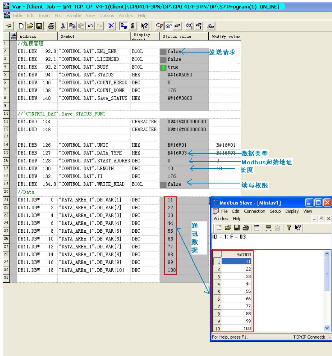
图 39:S7-400 单站系统 作为客户端与 Modbus Slave 软件通讯
