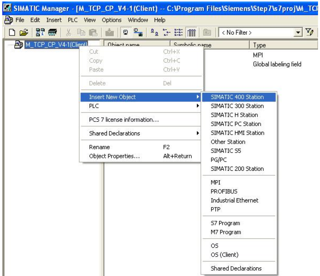
图 25:新建 S7-400 H Station
