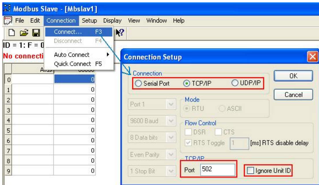
图 29:对应 TCP connection 的 Modbus Slave 连接窗口
