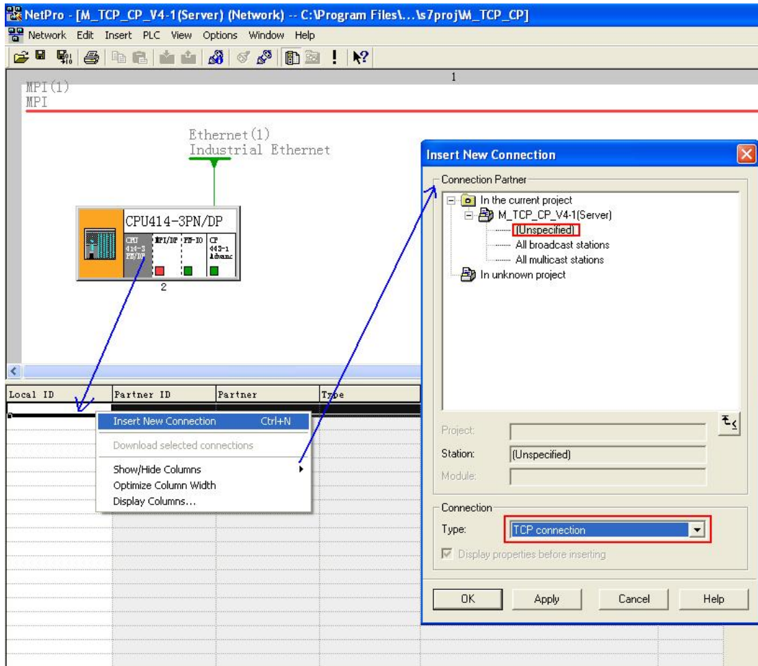
图 15:网络组态-新建 TCP connection
