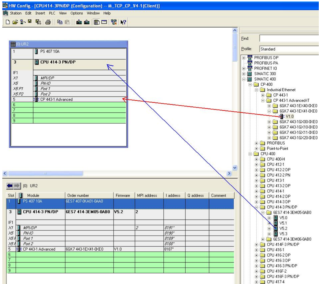
图 26: 硬件组态并设置 CP443-1 的 IP 地址
