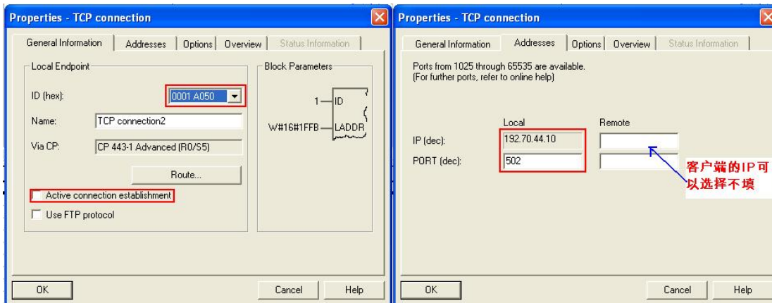
图 17:S7-400 为服务器的 TCP connection 参数设置
