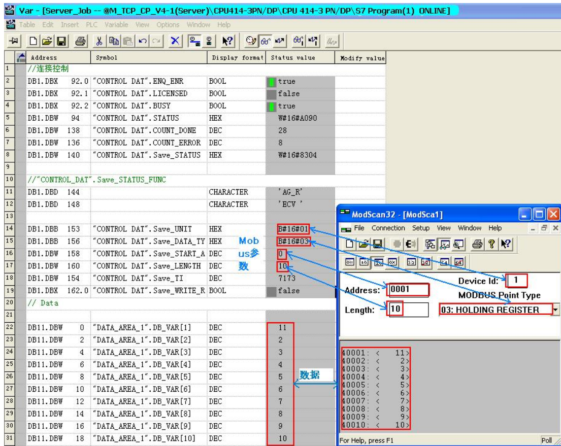
图 24:通讯连接建立
