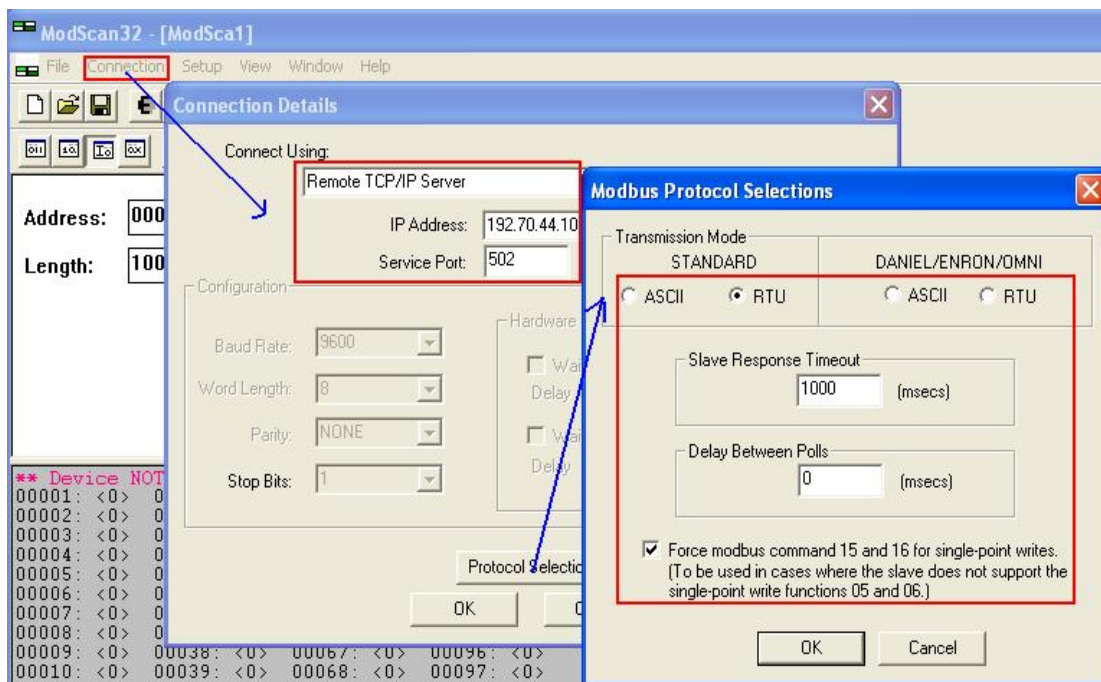
图 18:对应 TCP connection 的 Modscan32 连接窗口
