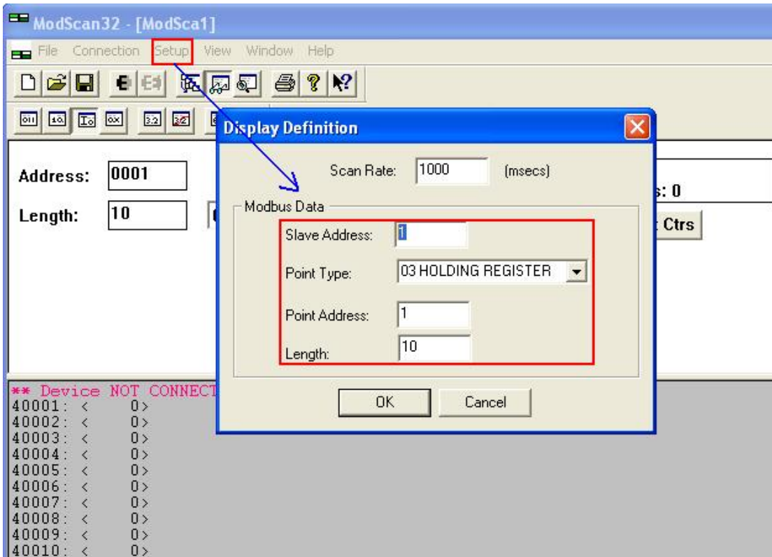
图 20:Modscan32 中 Modbus 数据参数定义
