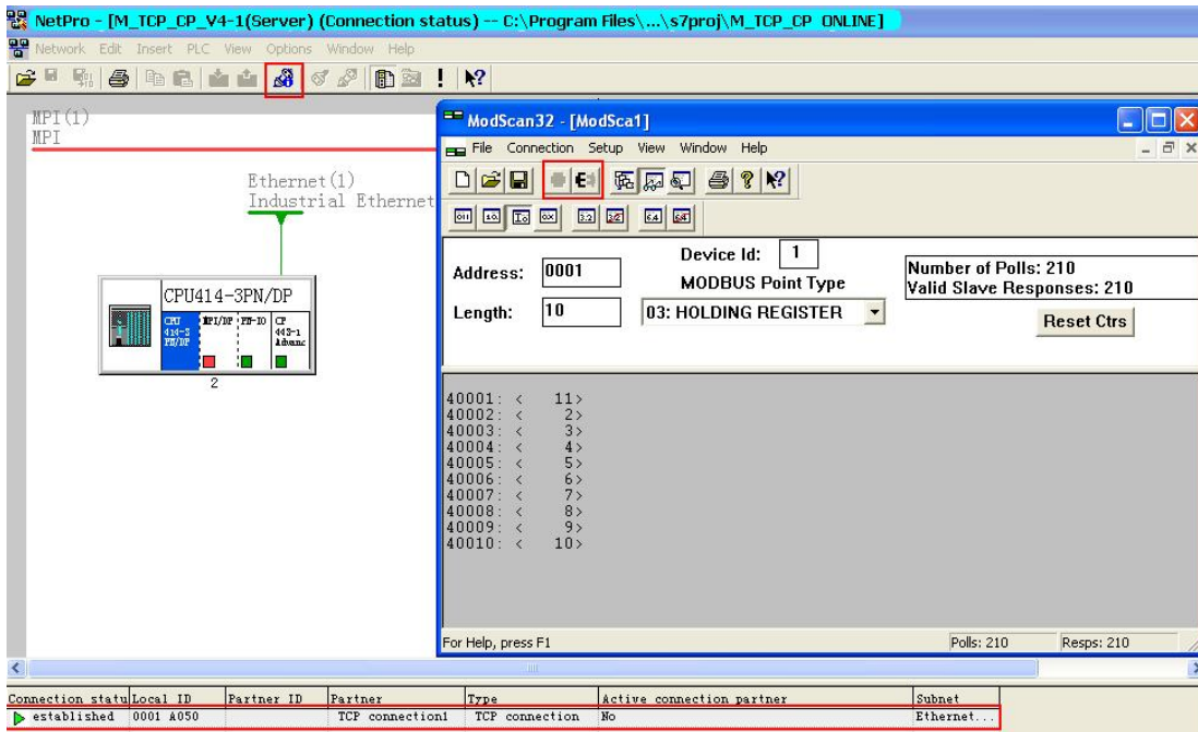
图 21: Modscan32 激活与 S7-400 的连接
