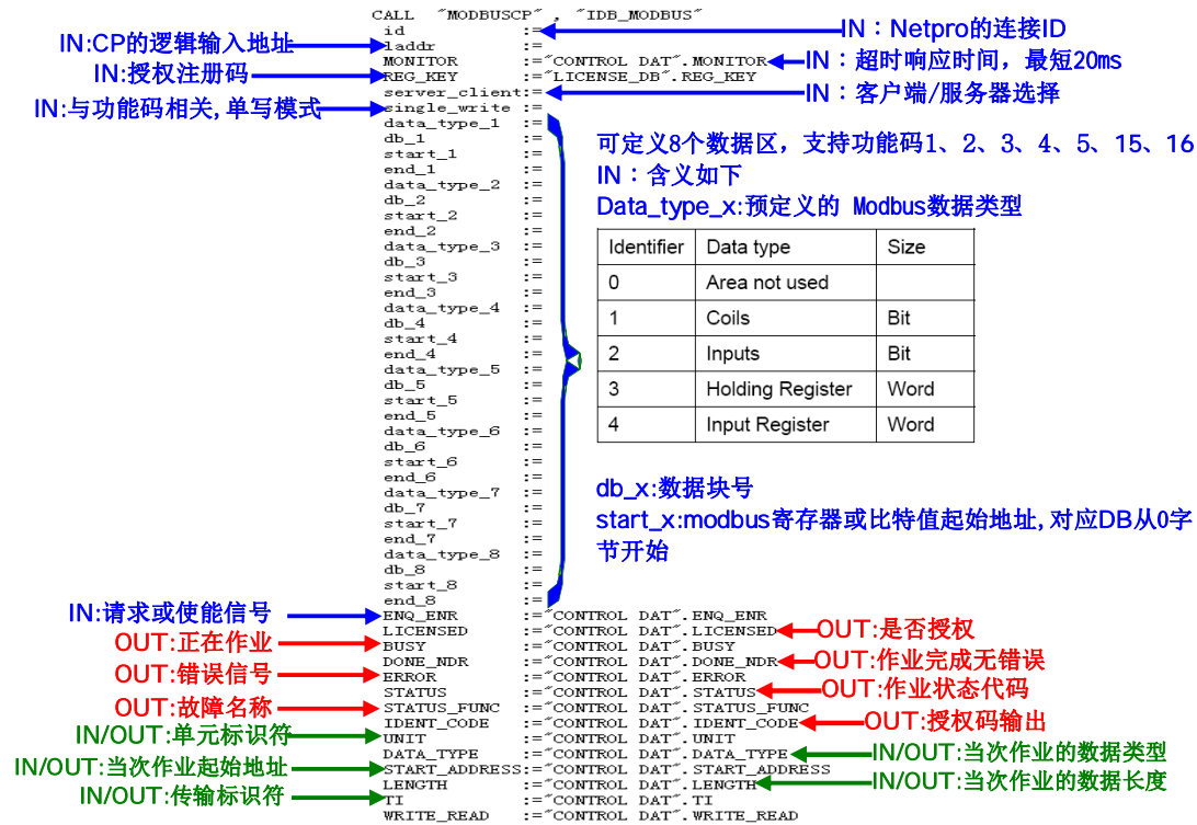
图 19: FB108“MODBUSCP”的管脚参数定义
