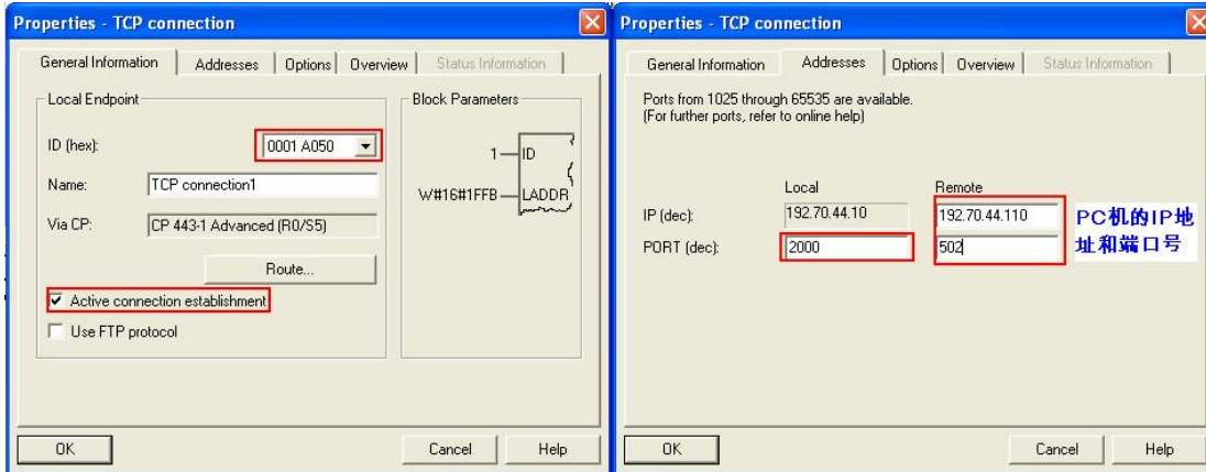
图 28: S7-400H 为客户端的 TCP connection1 参数设置
