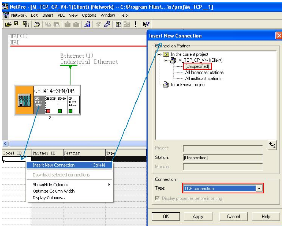
图 27: 网络组态-新建 TCP connection
